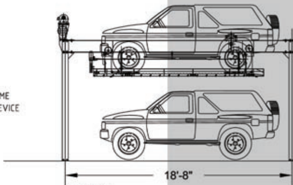
SP100 SIDE ELEVATION
